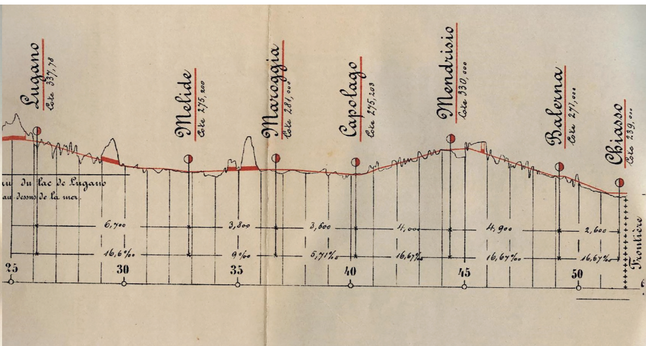
Figura 3. Profilo longitudinale della linea Lugano-Chiasso.
